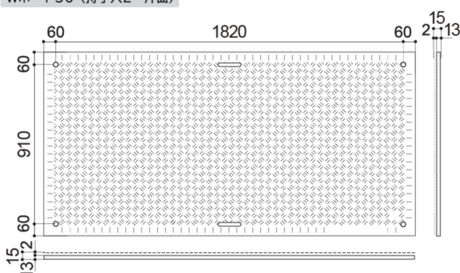
Wボード36 (持ち手穴2・片面)
