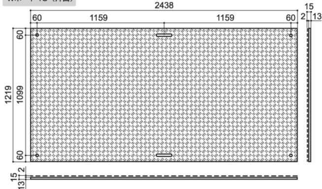
Wボード48 (片面)
